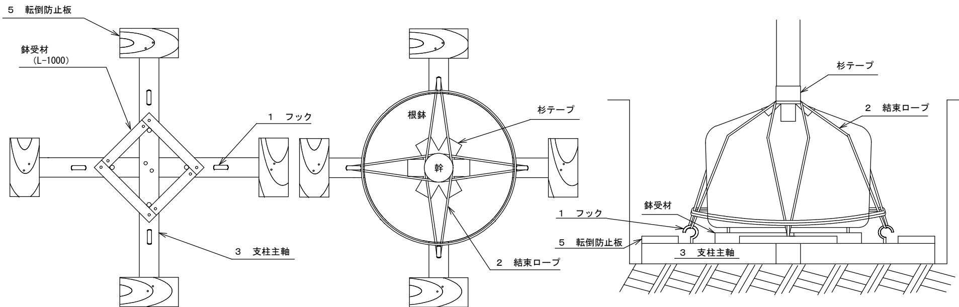
側面図
